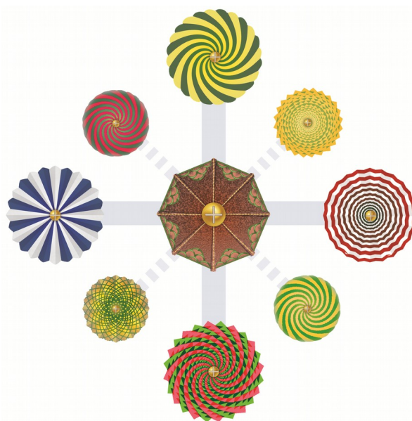
Исто коло као основа Покровског храма: кретање Мајке Земље - (крст од четири мале куполе) око Сунца (крст од четири велике куполе)
