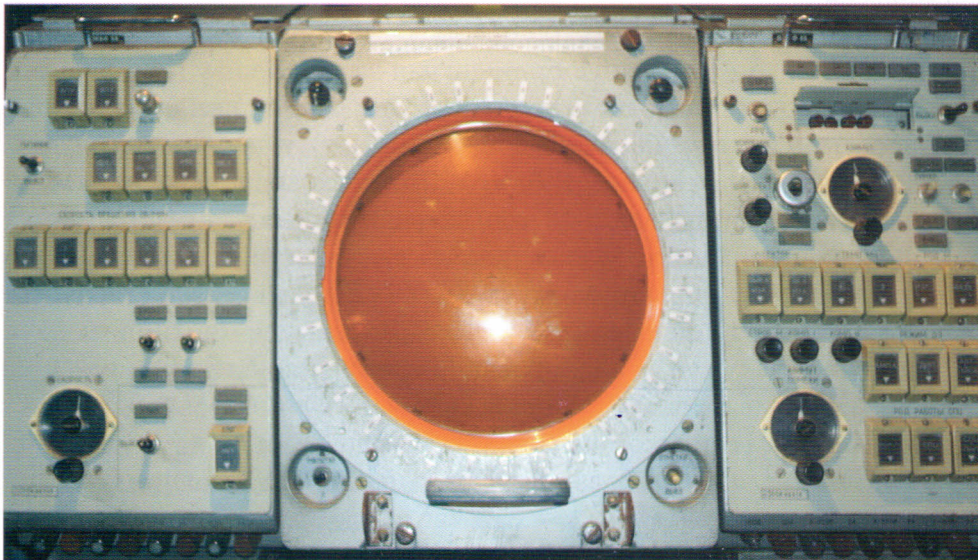
Показивач кружної осмайрања радара П-18 у кабини УНК (ВИКО)
